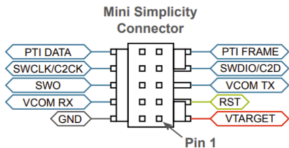
Figure 2.4. Mini Simplicity Connector
